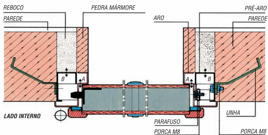
Vista interna dos perfis de remate e de fixação do revestimento interno na versão TOP
